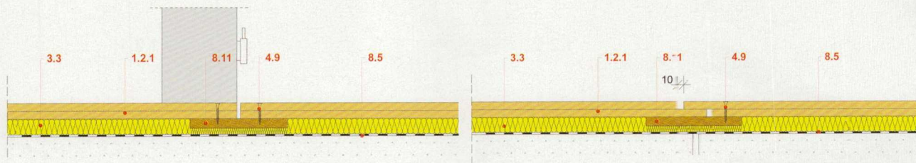
Küszöb kialakítás Rigidur szárazpadlóban
